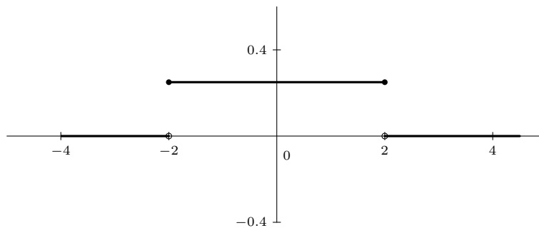
Slika 1: Funkcija gustoće vjerojatnosti f_X slučajne varijable X za a = -2 i b = 2 .
