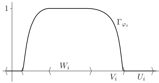
Graf funkcije \varphi_i
